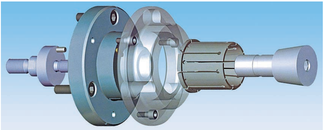
3 Hülsenspanndorn
