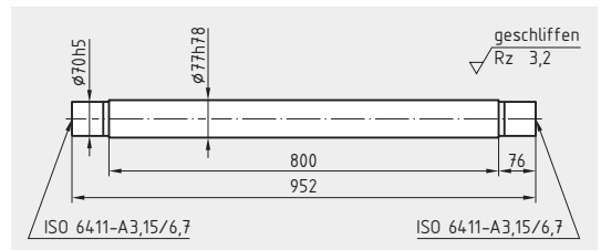
3 Getriebewelle
