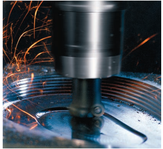
1 Spanende Fertigung
