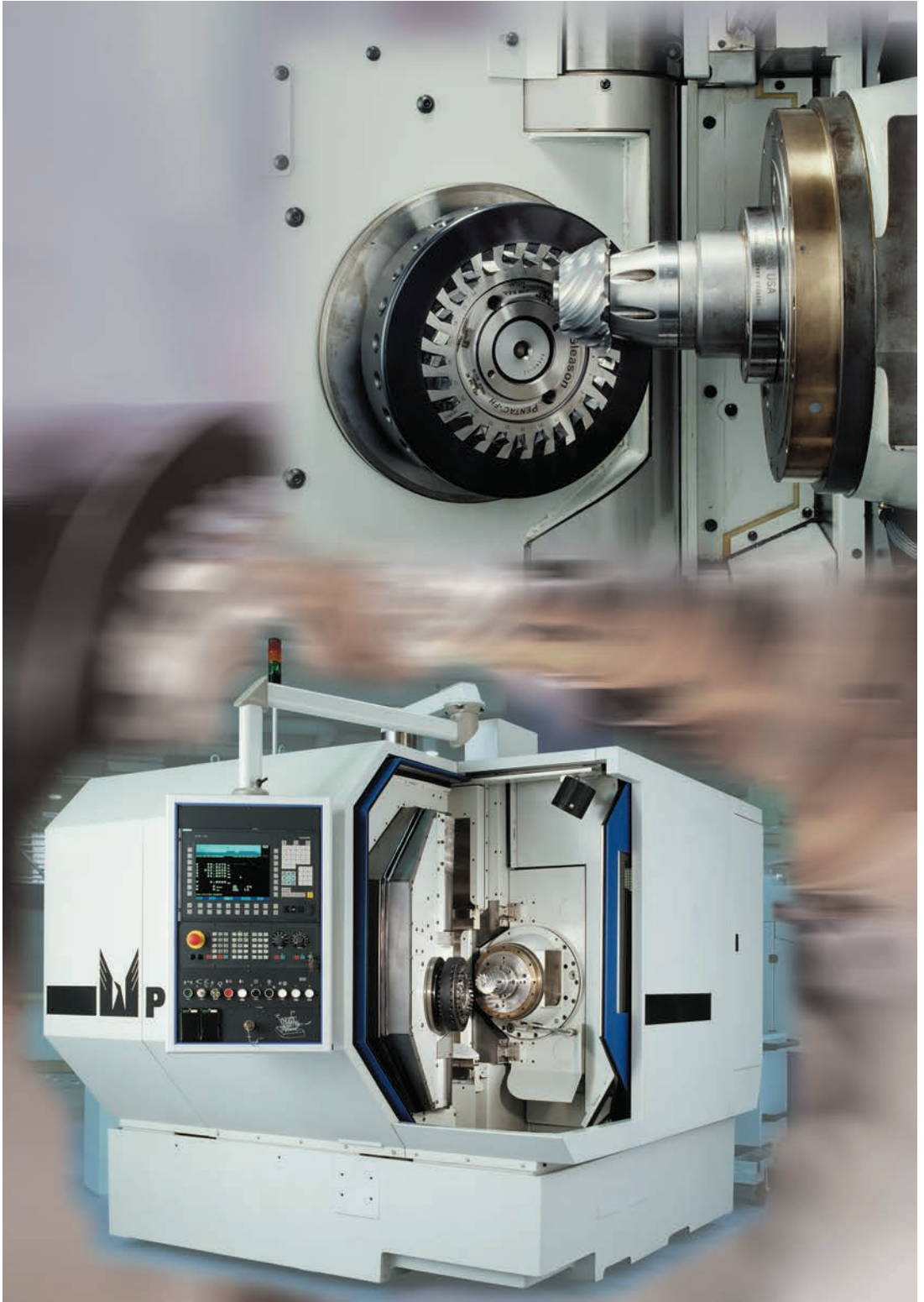
Kegelrad – Wälzfräsmaschine
